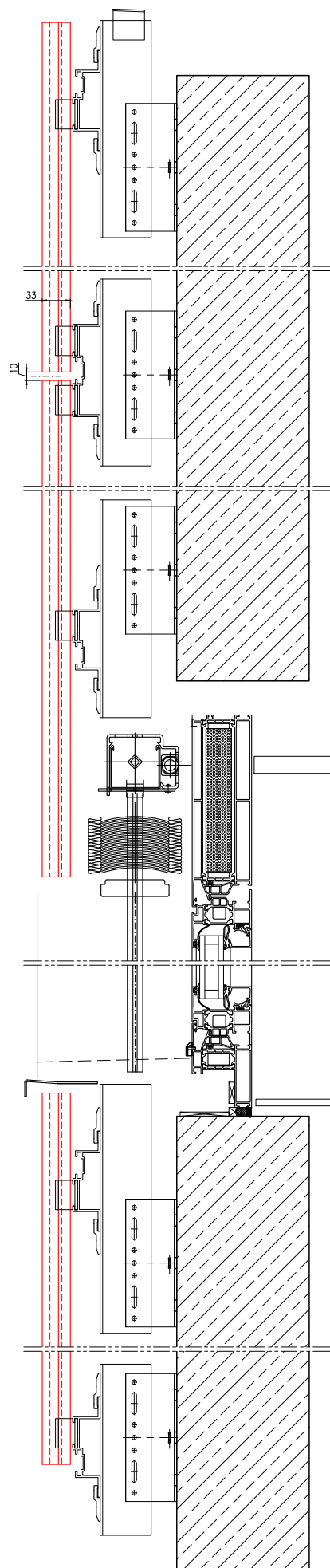
Schnitt A
