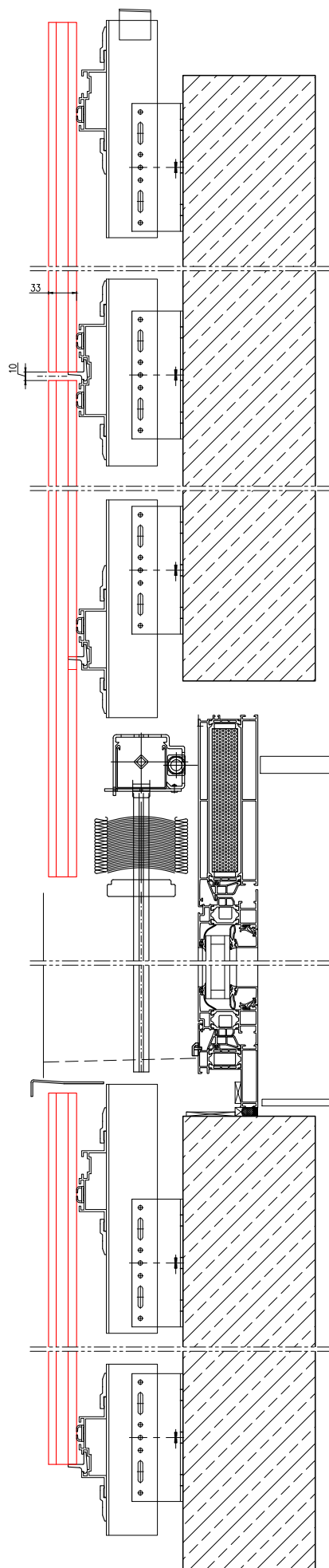
Schnitt B
