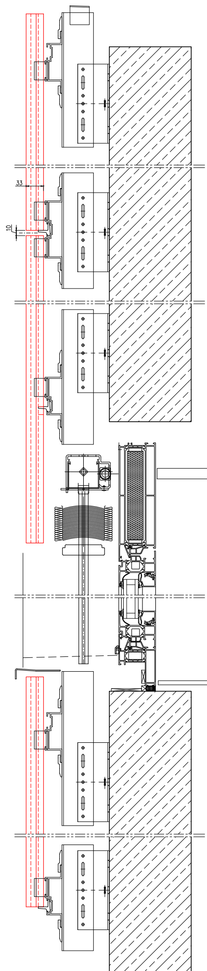
Schnitt A
