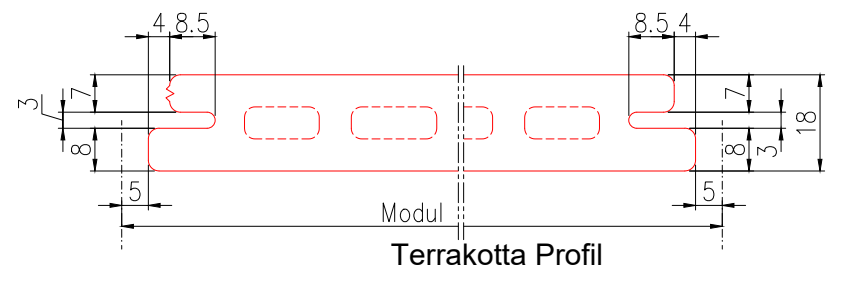
Einzelteile
