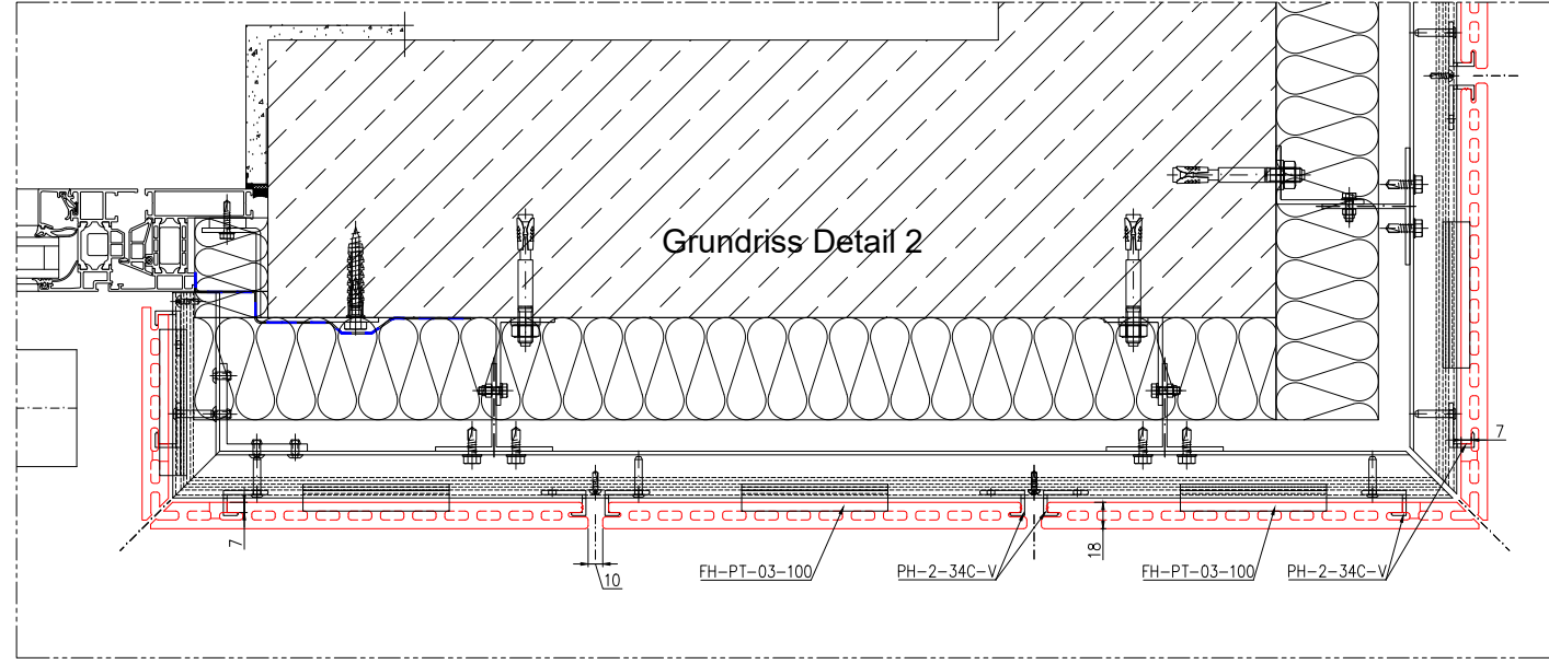
Terrakotta Profil
