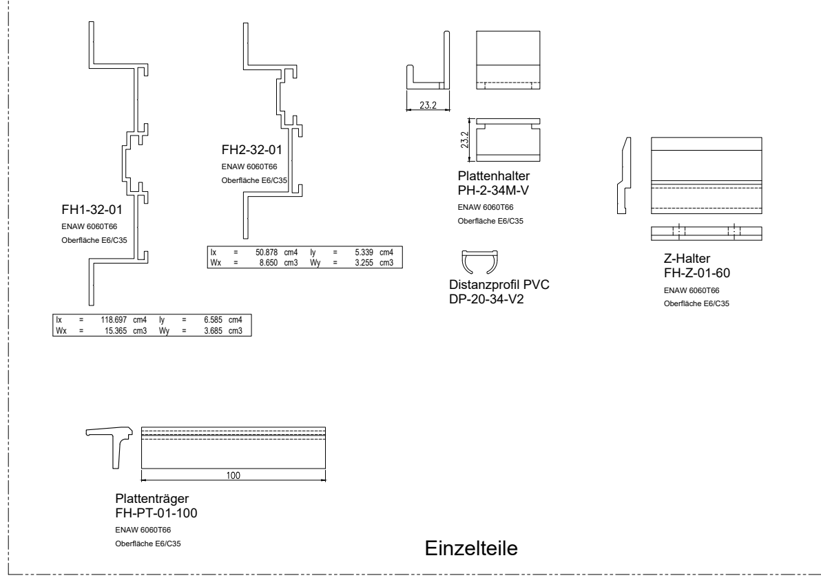
Variante horizontale Fuge Variante untere Abschluss Variante obere Abschluss
